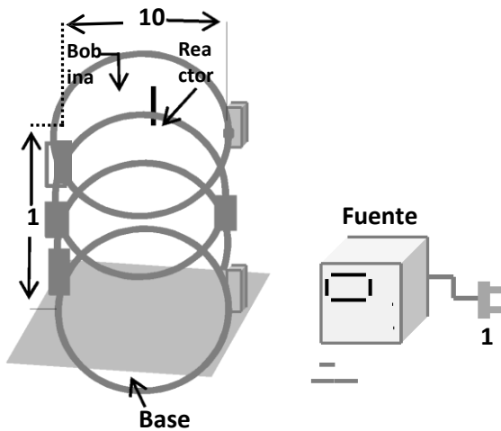
Figura 1. Bobina generadora de Campos Electromagnéticos
